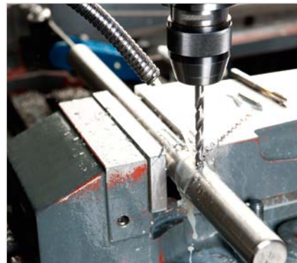
Bohren von Wellen
