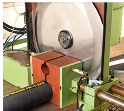
Millimetergenaues Ablängen
