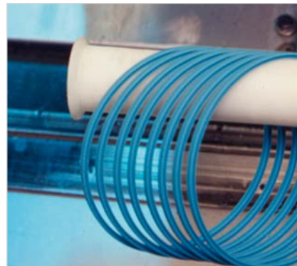
Expressfertigung – mechanische Produktion von Dichtungen
