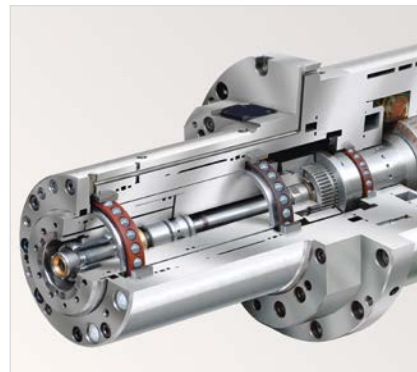
Spindelservice
