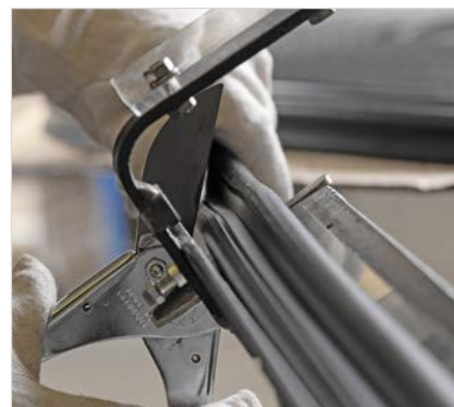
Profile ablängen
