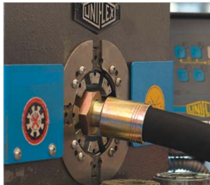
Montage Hydraulikschlauchleitungen
